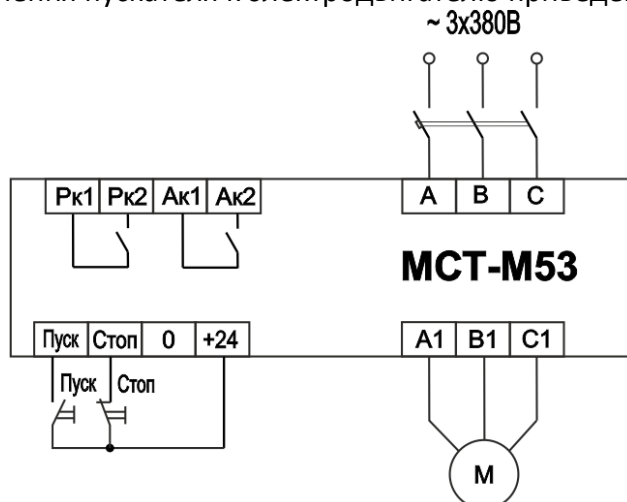
Рисунок 4 – Пример схемы подключения ЭД
